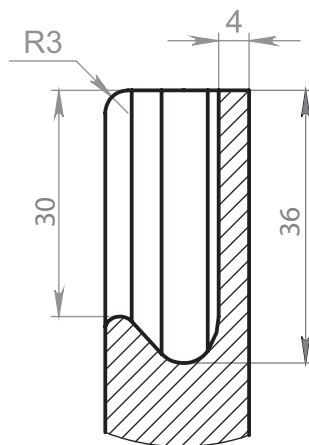
Вид ручки в разрезе
